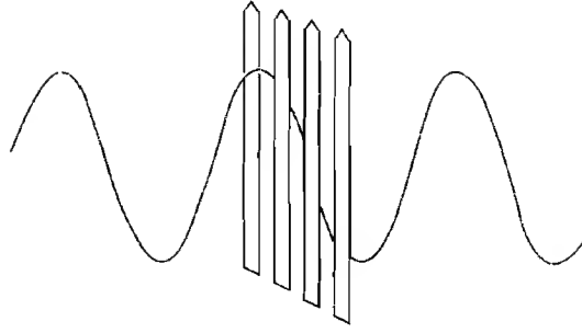
شكل ١٠-١: موجات مستقطبة رأسياً تمرق عبر «ألواح السور».
